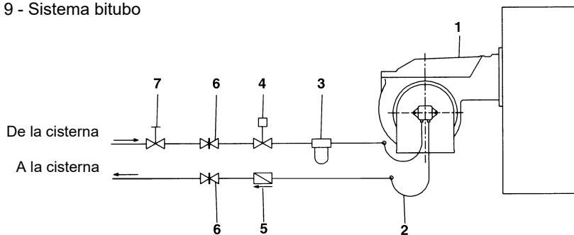
Fig. 9 - Sistema bitubo
