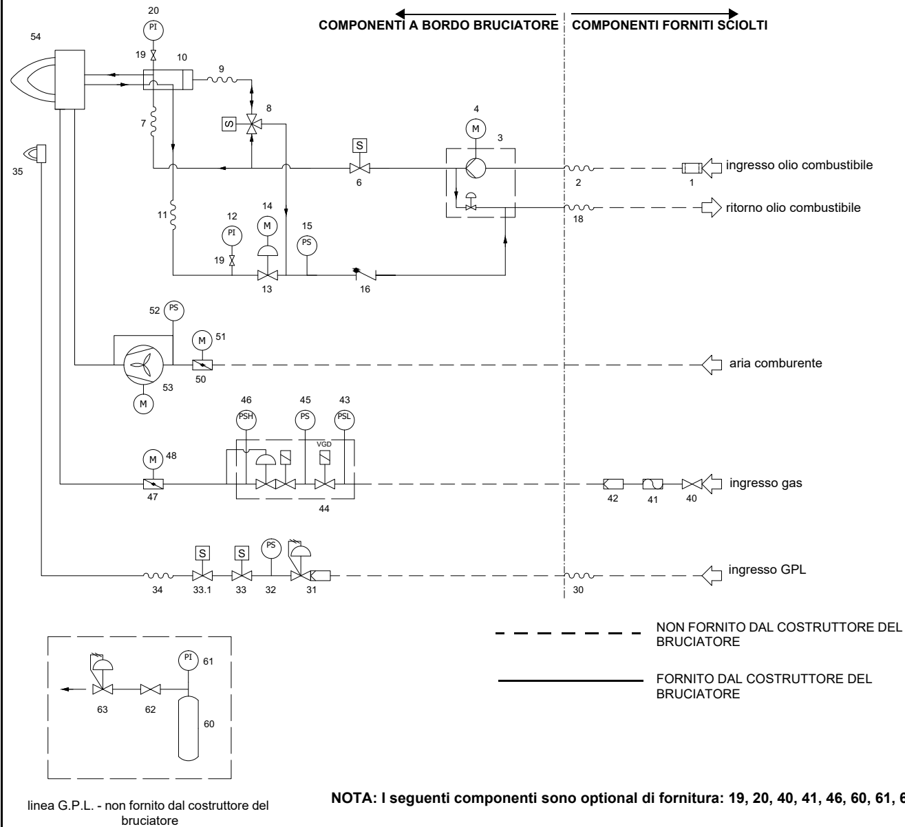
Fig. 4 - 3I2MG-19 v0 Schema idraulico - ugello tipo M3
