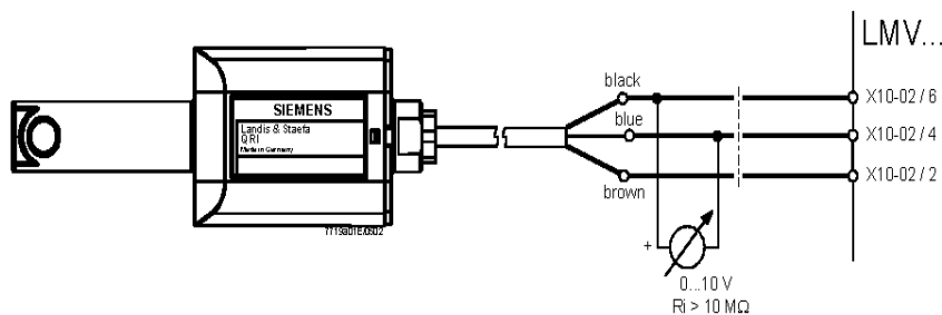
Fig. 13 - Rilevazione con fotocellula QRI..
