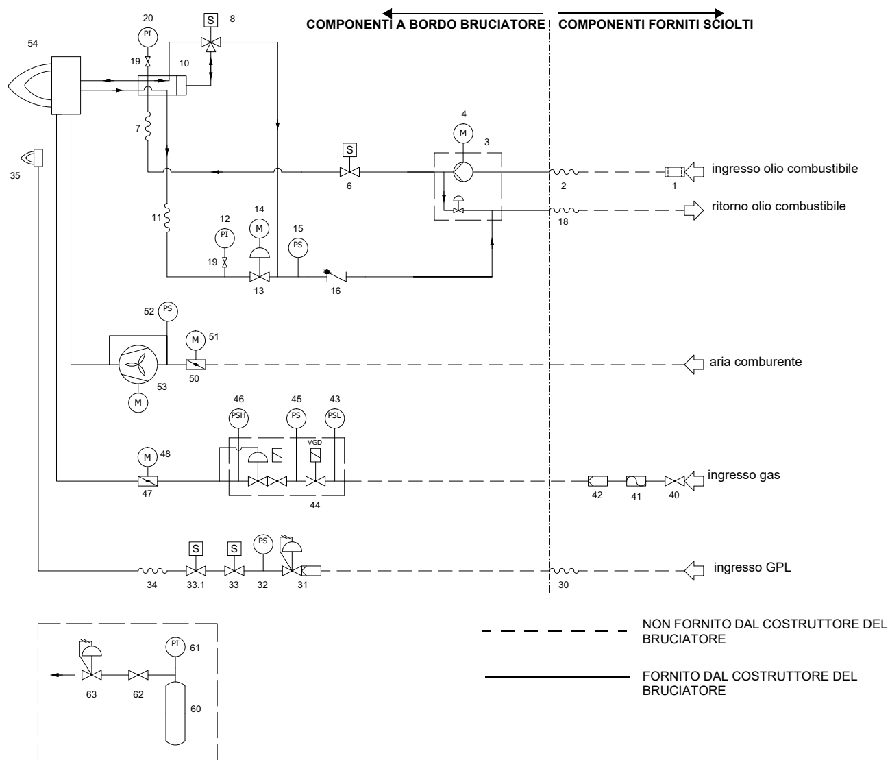
Fig. 5 - 3I2MG-20 v0 Schema idraulico - ugello tipo G, KV
