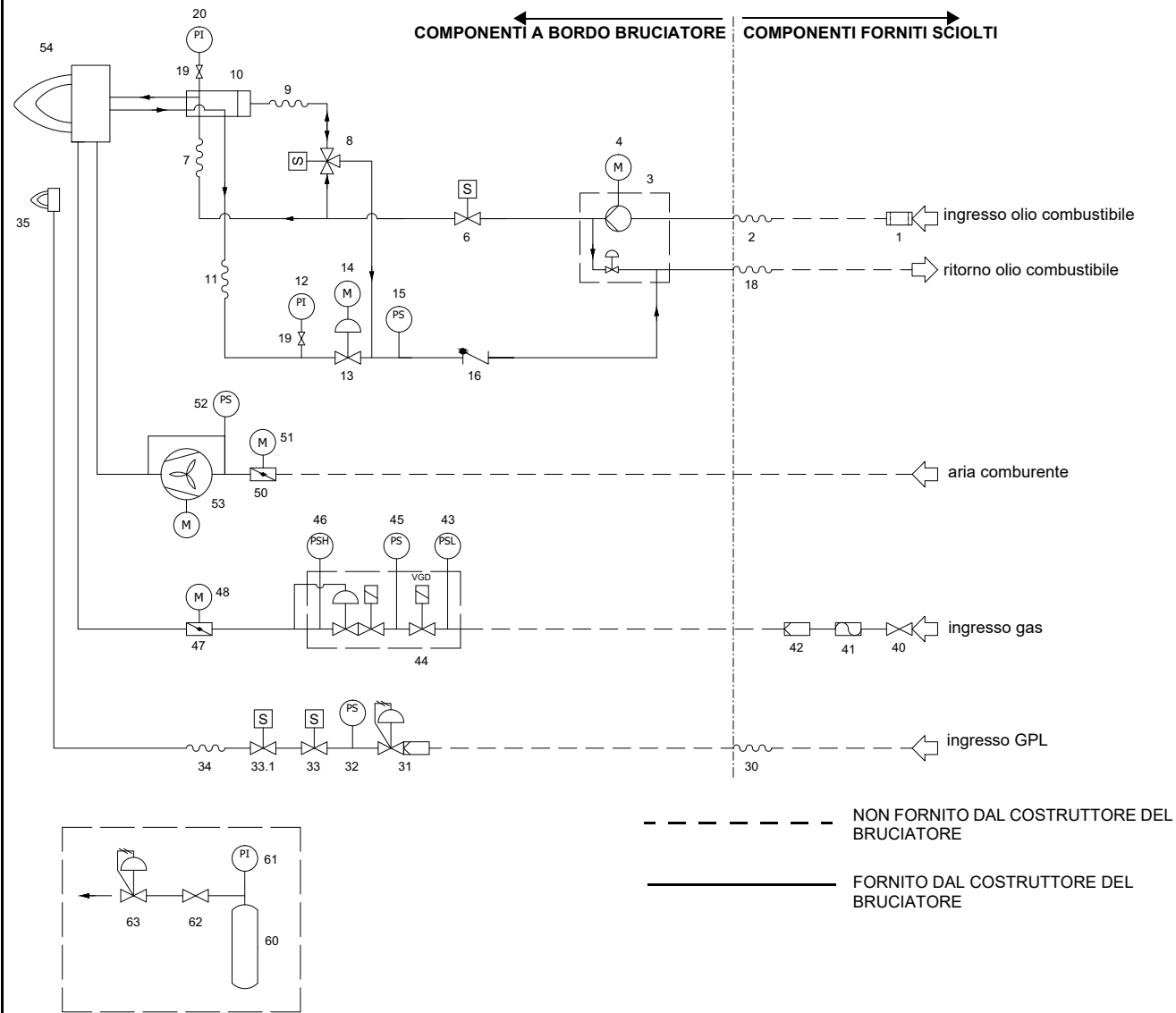
Fig. 4 - 3I2MG-19 v0 Schema idraulico - ugello tipo M3
