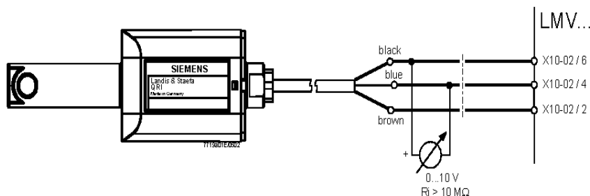
Fig. 13 - Rilevazione con fotocellula QRI..
