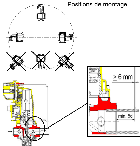
SIEMENS VGD.. Positions de montage
