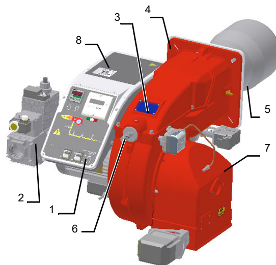
Горелка с алюминиевым воздухозаборником
