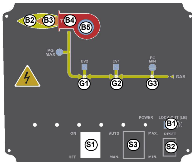
Рис. 3: передняя панель электрощита горелки
