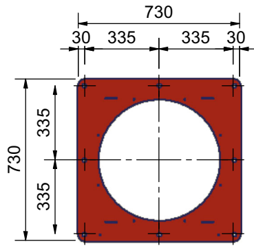
фланец горелки
