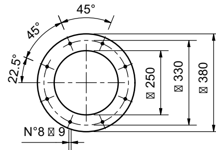
фланец FGR
