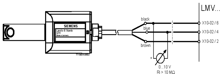
Рис. 7 - Детектирование с фотоэлементом QRI..
