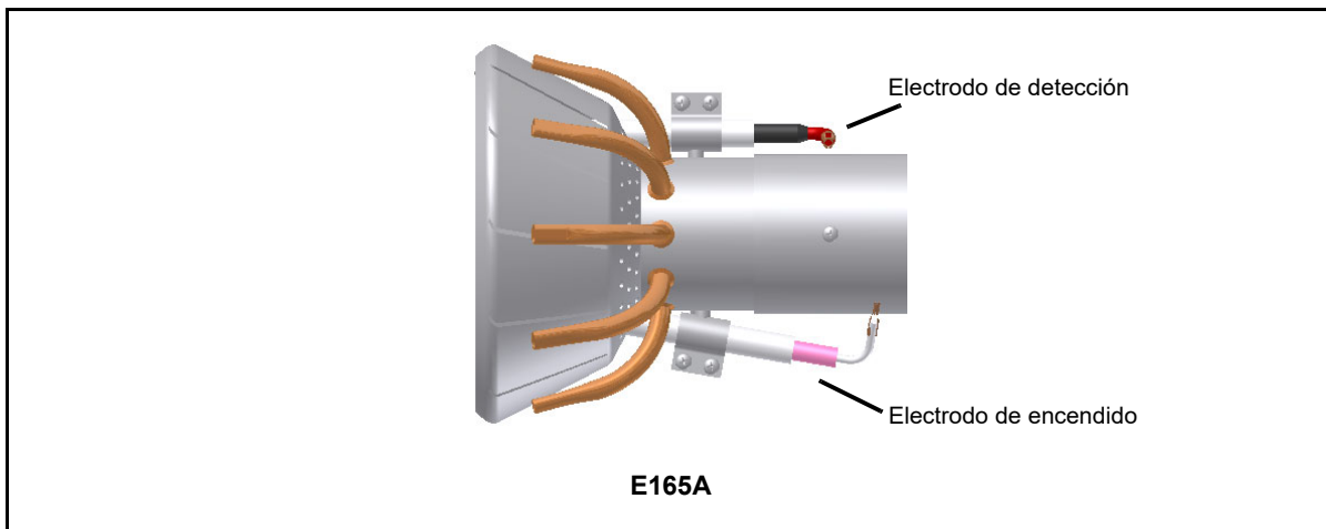
Regulación de la posición de los electrodos (quemador piloto, si está previsto)
