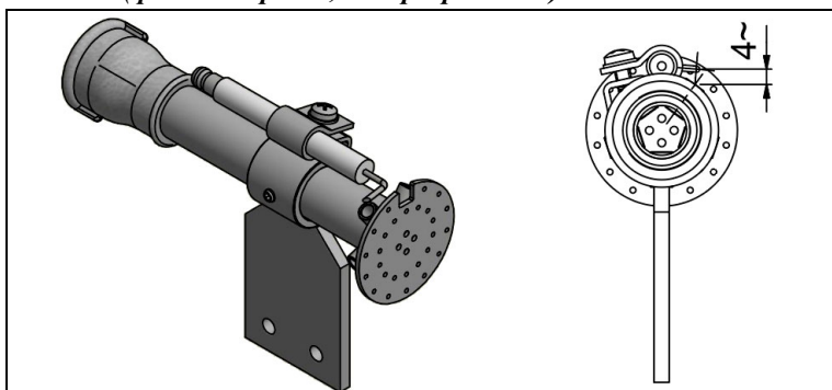
Regulación de la posición del electrodo (quemador piloto, si se proporciona)
