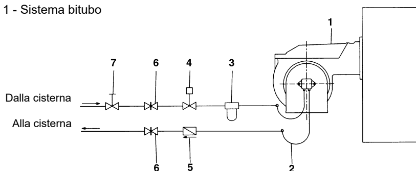
Fig. 1 - Sistema bitubo
