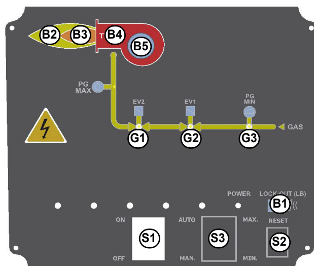
Fig. 3 Panel frontal cuadro eléctrico
