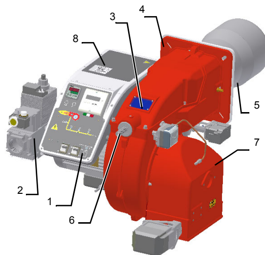
Quemador con caja aspiración de aire en aluminio
