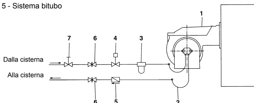
Fig. 5 - Sistema bitubo
