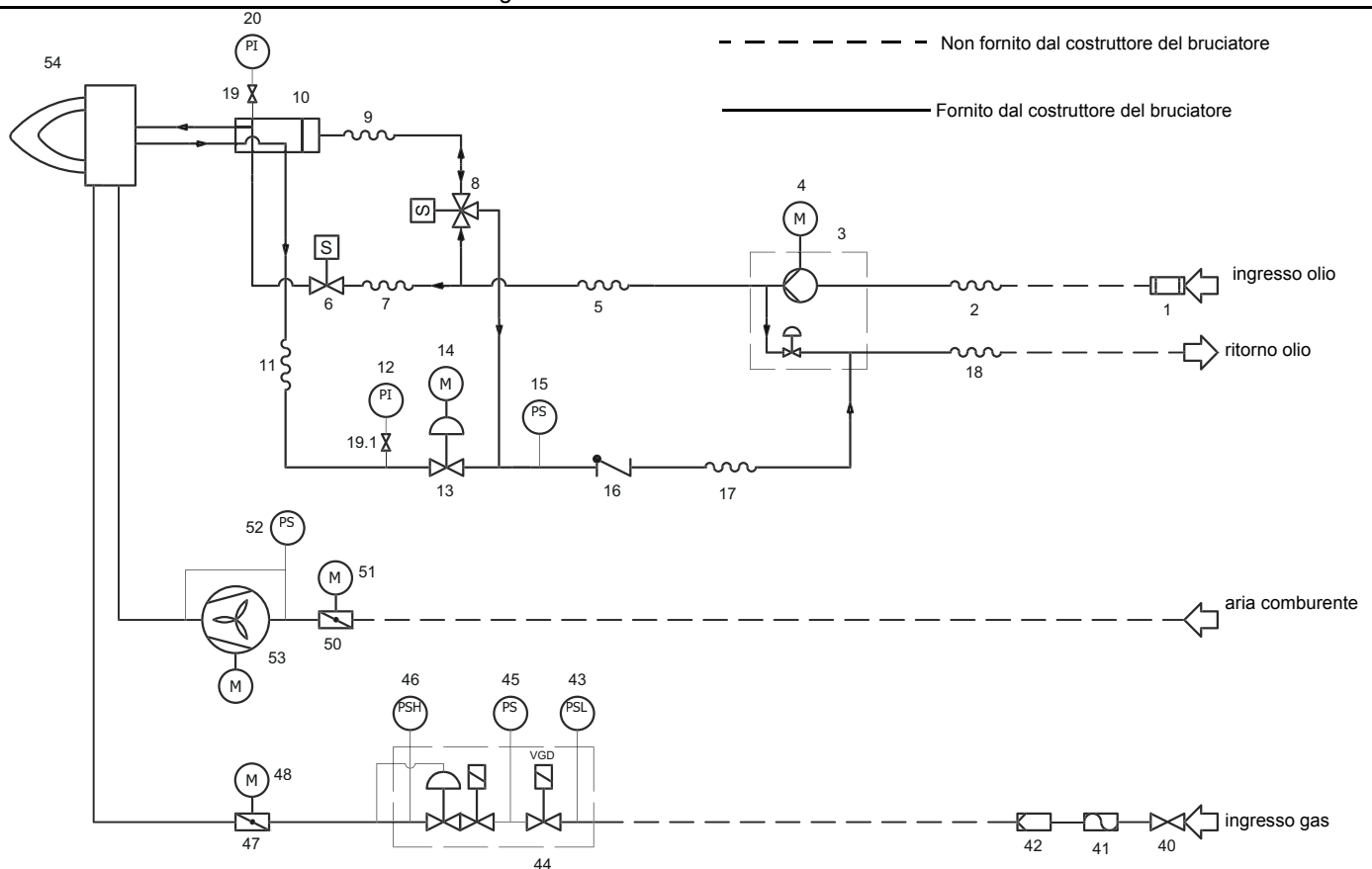
Fig. 4 - 3I2MG-23 v0 Schema idraulico
