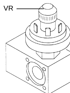
Fig. 23 - Pressostato SIT
