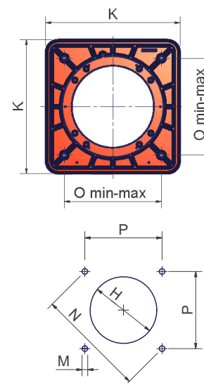
Рекомендуемая амбразура котла
