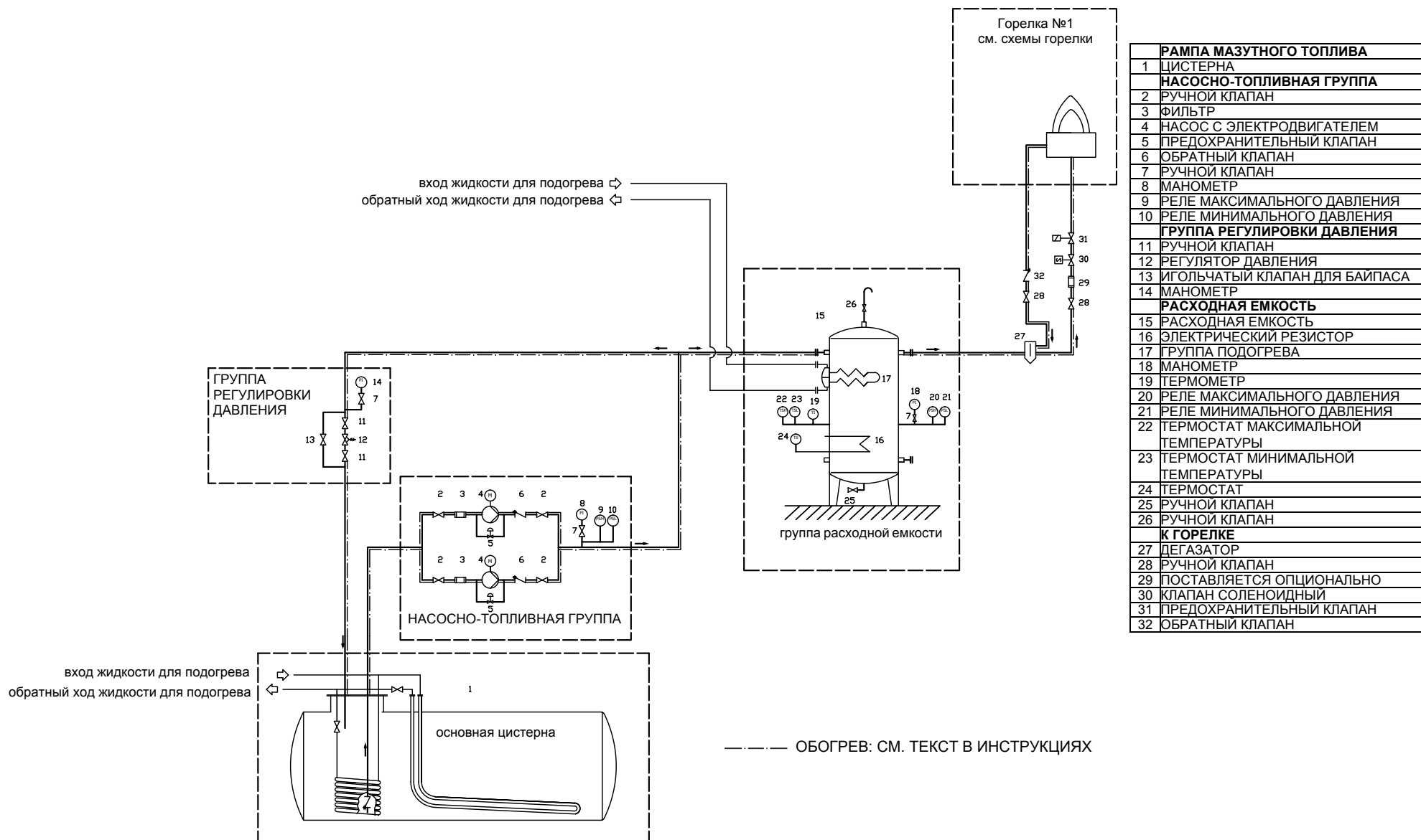
Рис. 10 - 3ID0023 v2 – Система подачи мазута при наличии одной горелки - Гидравлическая схема
