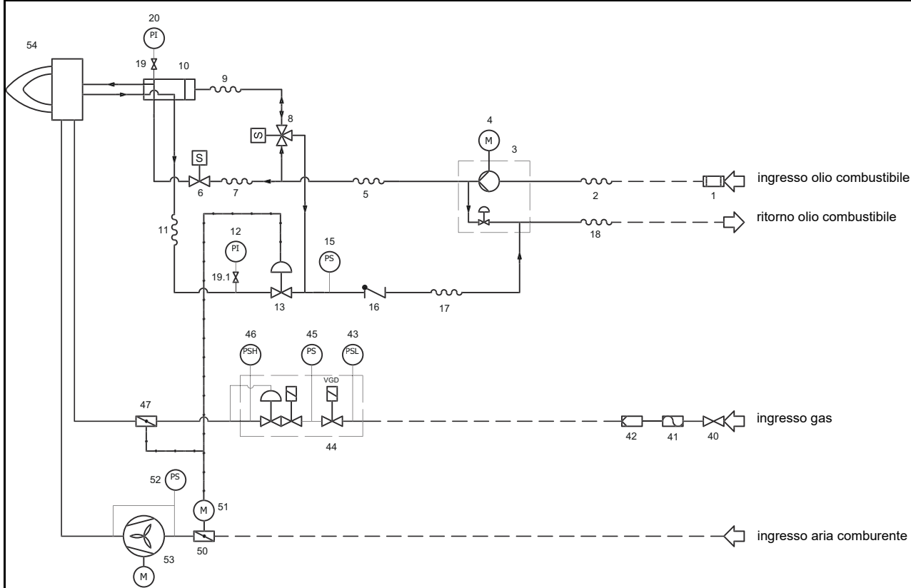
Fig. 4 - 312MG-24 v0 Schema idraulico
