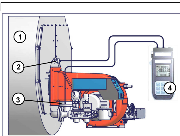
Ориентировочный чертеж.Описание
