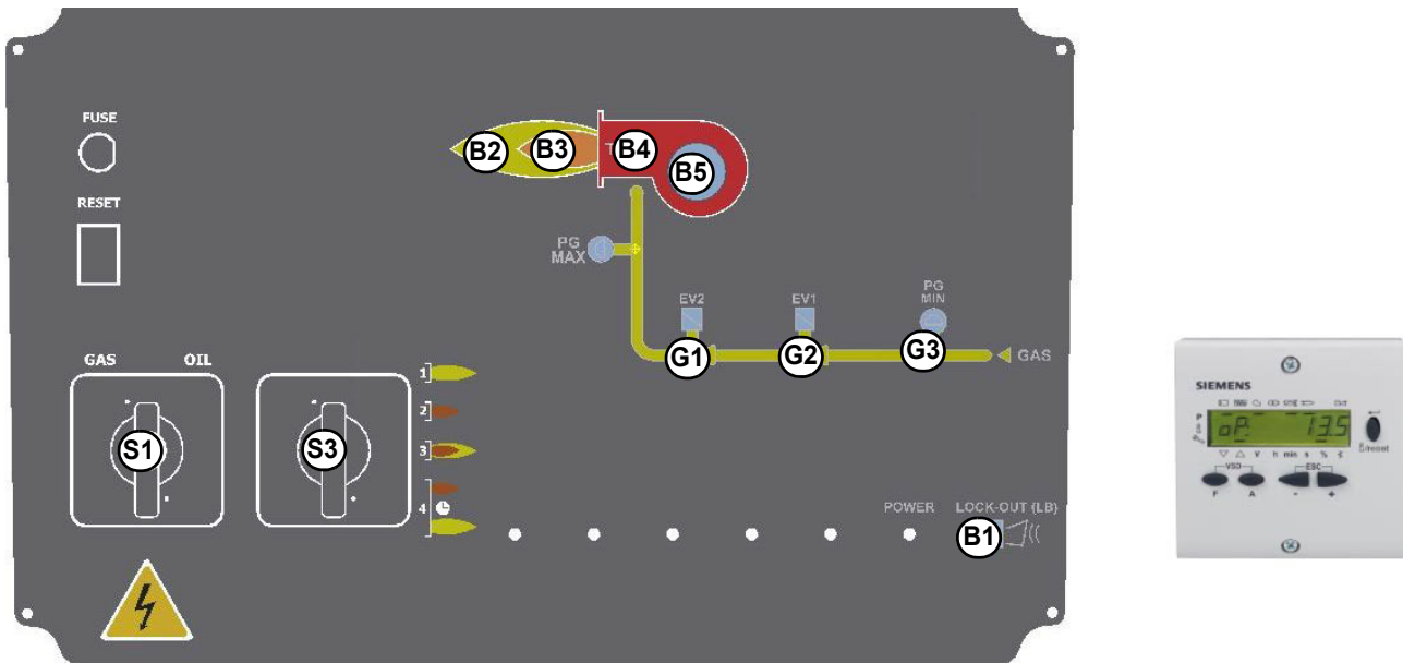
Рис. 4: передняя панель электрошита горелки
