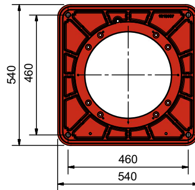
Фланец горелки
