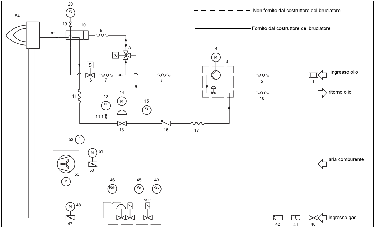
Fig. 4 - 3I2MG-23 v0 Schema idraulico
