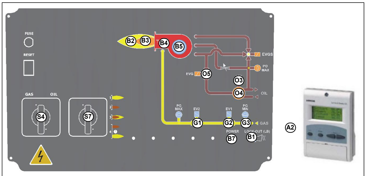
Fig. 4 - Pannello frontale quadro elettrico bruciatore
