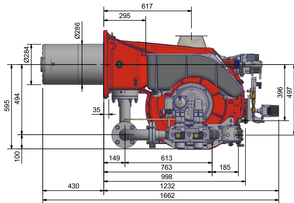
flangia FGR
