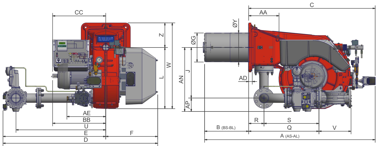
Flangia bruciatore
