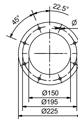
flangia FGR
