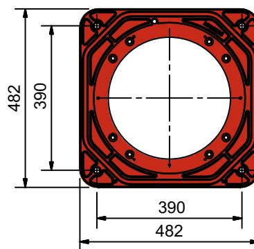
Flangia bruciatore
