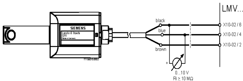
Fig. 8 - Rilevazione con fotocellula QRI..
