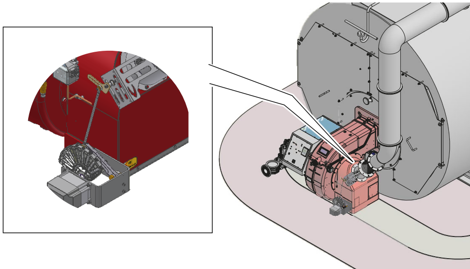
Serranda FGR (ricircolo fumi) su bruciatore
