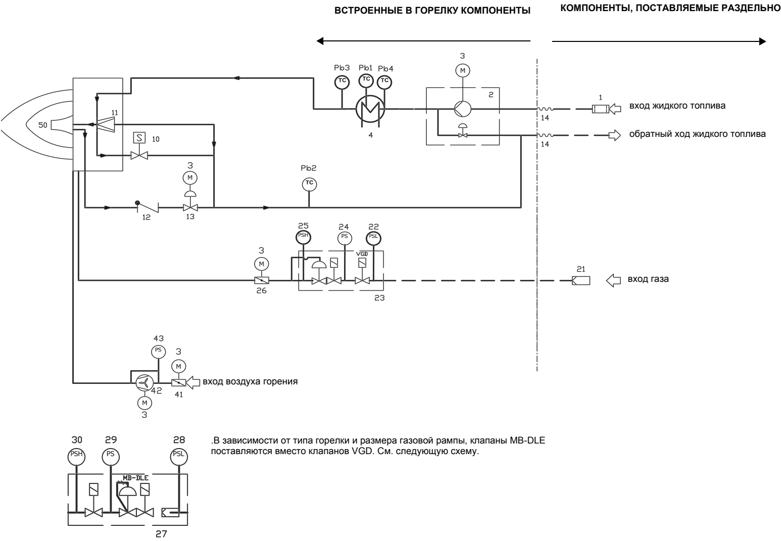
Рис. 2 Гидравлическая схема 3I2MD24 v1
