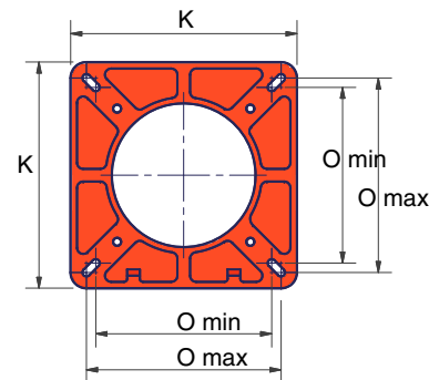
Фланец горелки
