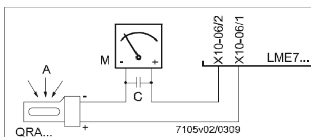
Fig. 16: Rilevazione con fotocellula QRA..
