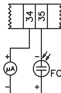
Fig. 14: Rilevazione con fotocellula QRA..
