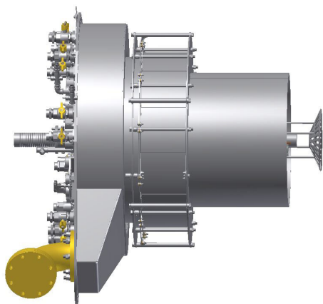
Газовый тор для распределения газа и группа газовых фурм, которые подлежат монтажу на воздушном коробе.
