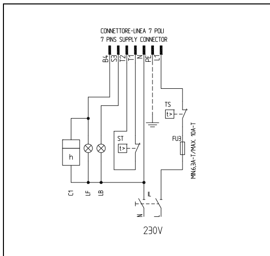
Connettore 7 poli
