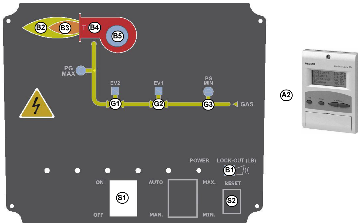
Рис. 6: передняя панель электрощита горелки
