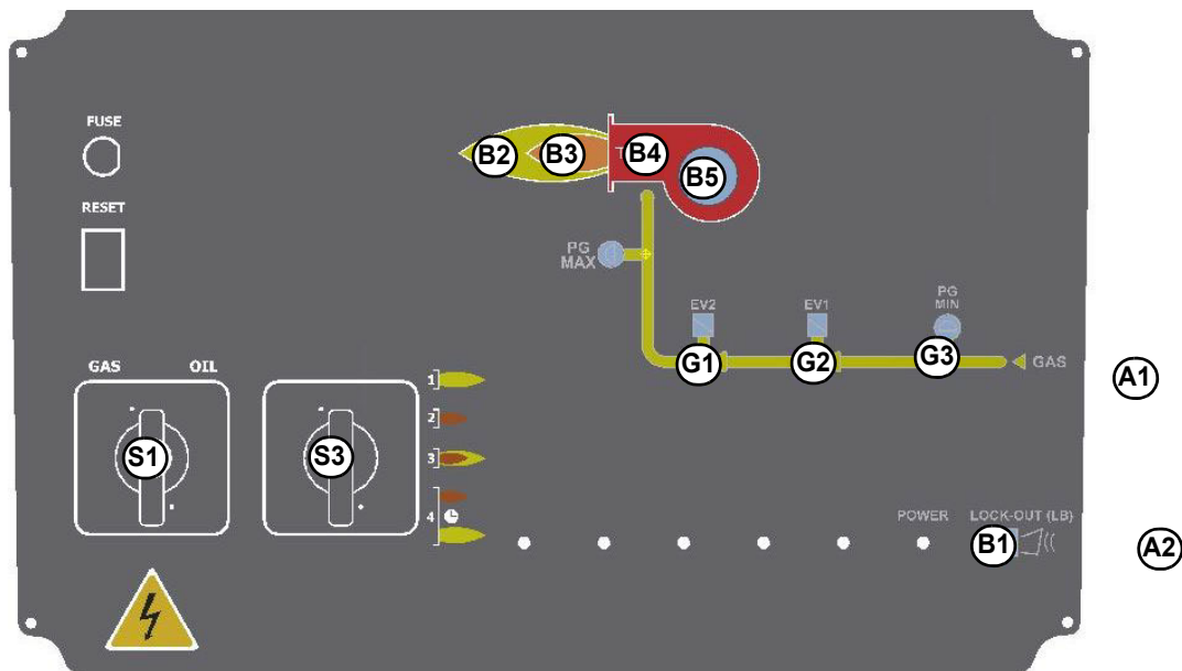
Fig. 6 Panel frontal cuadro eléctrico
