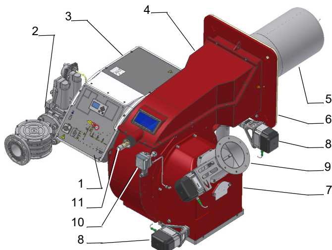
Esempio di bruciatore con FGR
