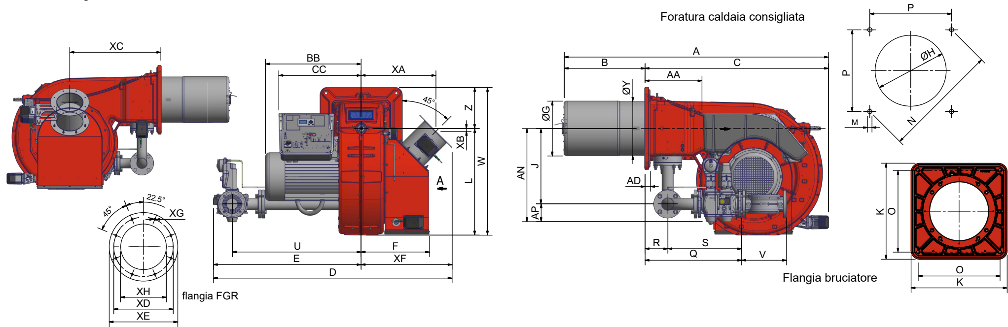
Dimensioni di ingombro in mm - versione con FGR
