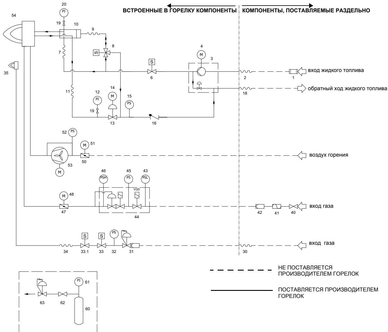
Рис. 1 - 3I2MG-19 v0 – Гидравлическая схема для форсунки типа МЗ
