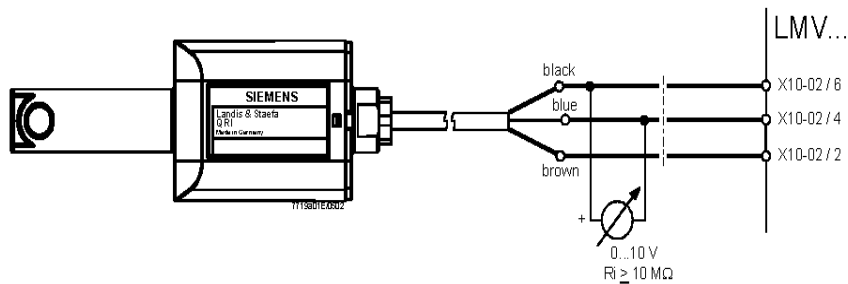
Рис. 14 - Детектирование с фотоэлементом QRI..
