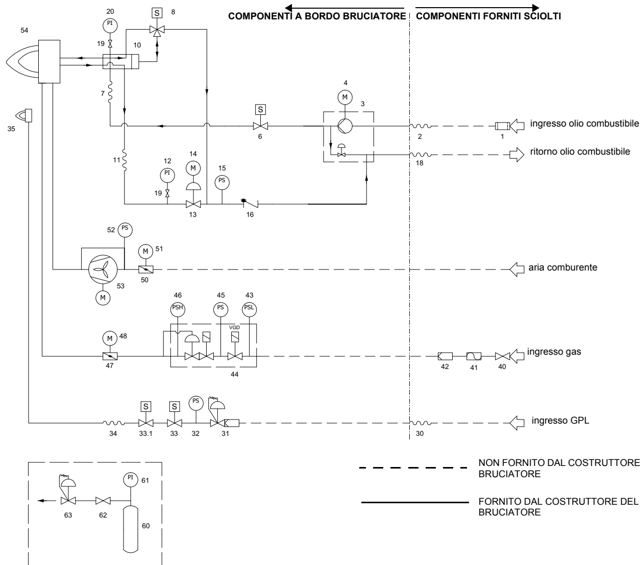
Fig. 2 - 3I2MG-20 v0 Schema idraulico - ugello tipo G, KV
