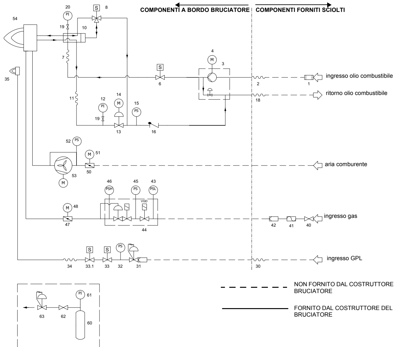
Fig. 2 - 3I2MG-20 v0 Schema idraulico - ugello tipo G, KV
