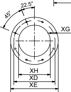
Flangia FGR
