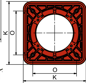
Flangia bruciatore
