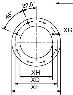
Flangia FGR
