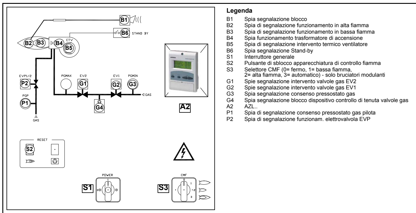
Fig. 6 - Pannello quadro elettrico
