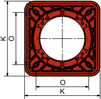
Flangia bruciatore
