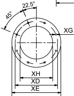
Flangia FGR
