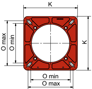
Flangia bruciatore
