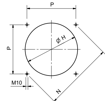
Foratura caldaia consigliata
