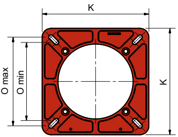
flangia bruciatore
