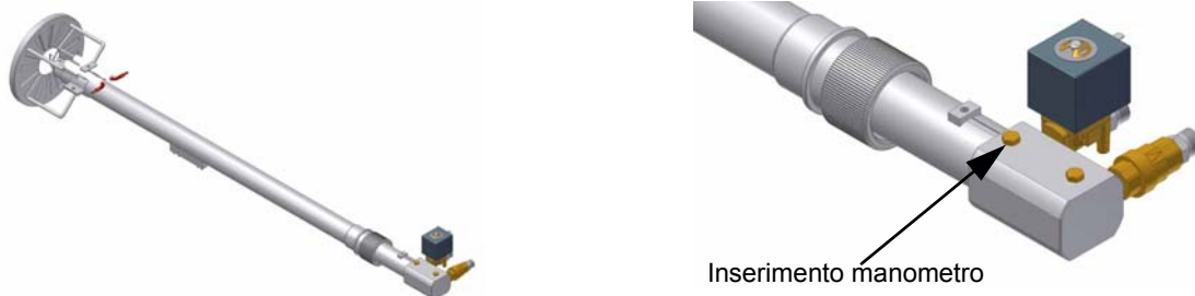
Fig. 15 - Testa di combustione con lancia gasolio (PG70 - PG81)
