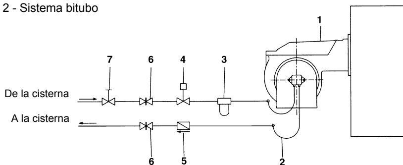
Fig. 2 - Sistema bitubo
