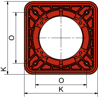
Фланец горелки
