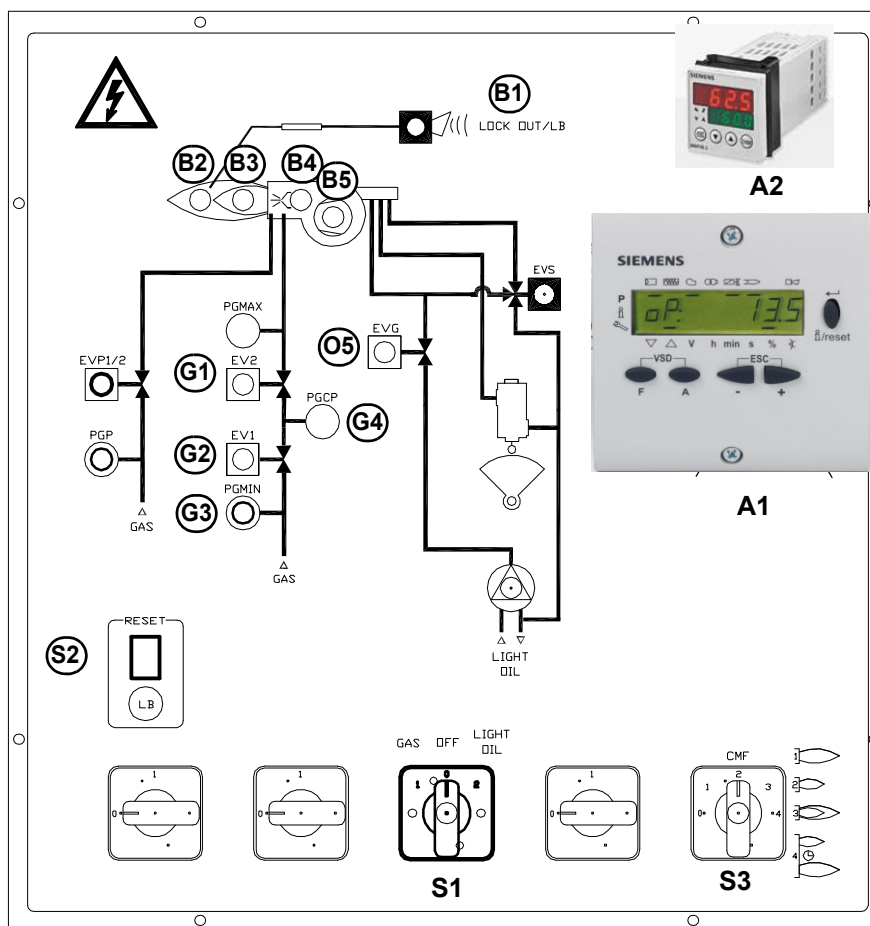
Рис. 6 - Лицевая панель электрощита
