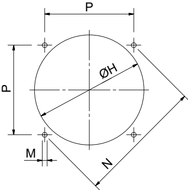
Схема сверления плиты котла
