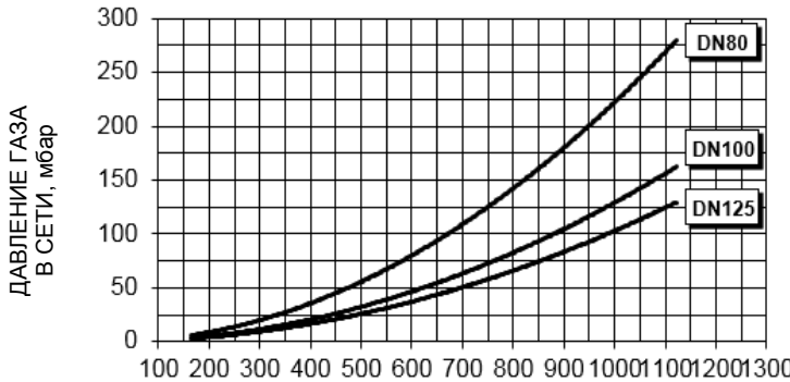
РАСХОД ГАЗА Стм³/час
