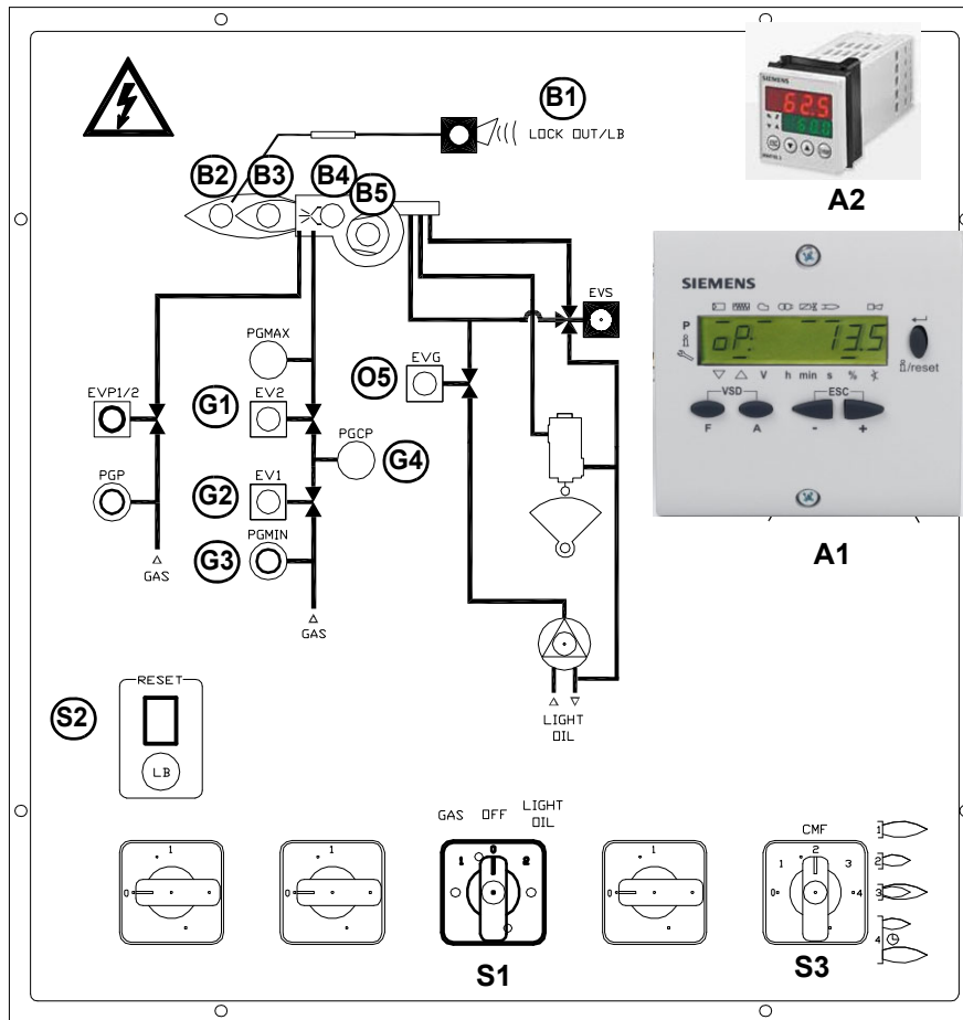
Рис. 6 - Лицевая панель электроцита
