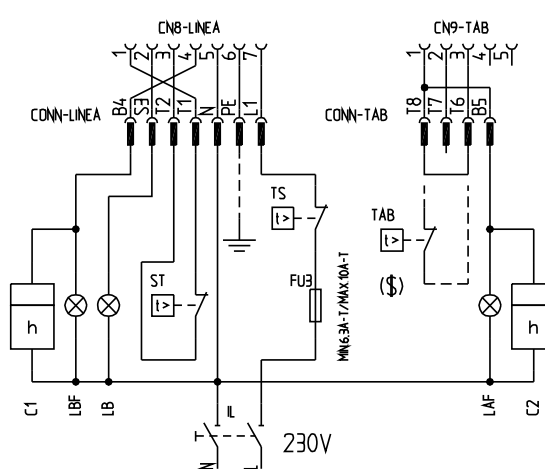
Fig. 20: Bruciatori bistadio
