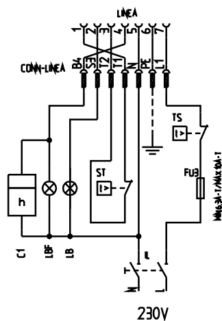
Fig. 19: Bruciatori monostadio
