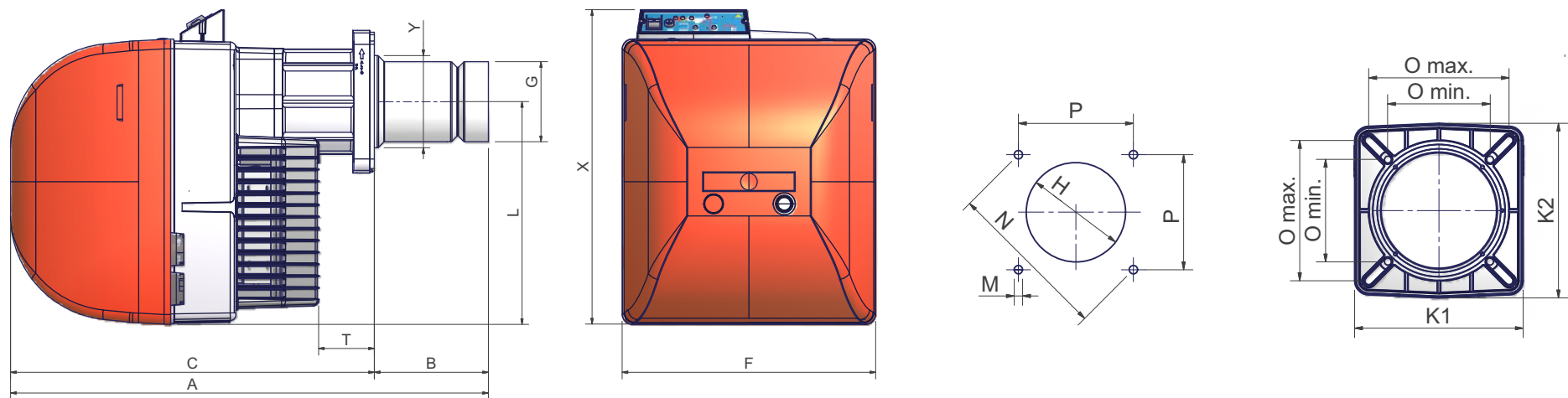
Foratura caldaia consigliata e flangia bruciatore
