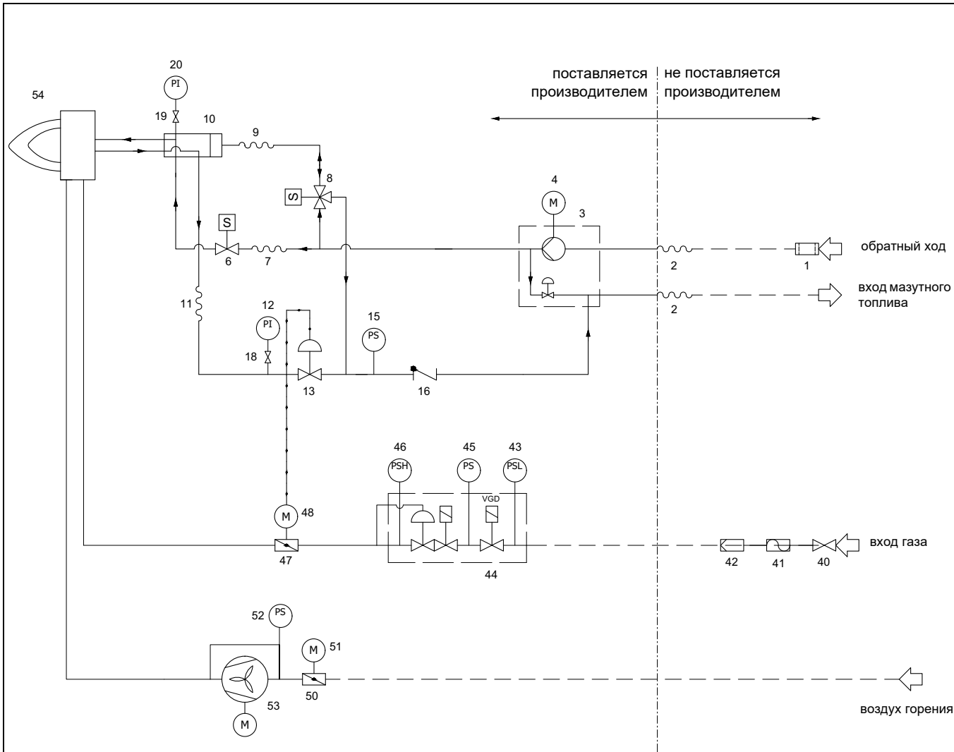
Рис. 1 3I2MG77 - Гидравлическая схема
