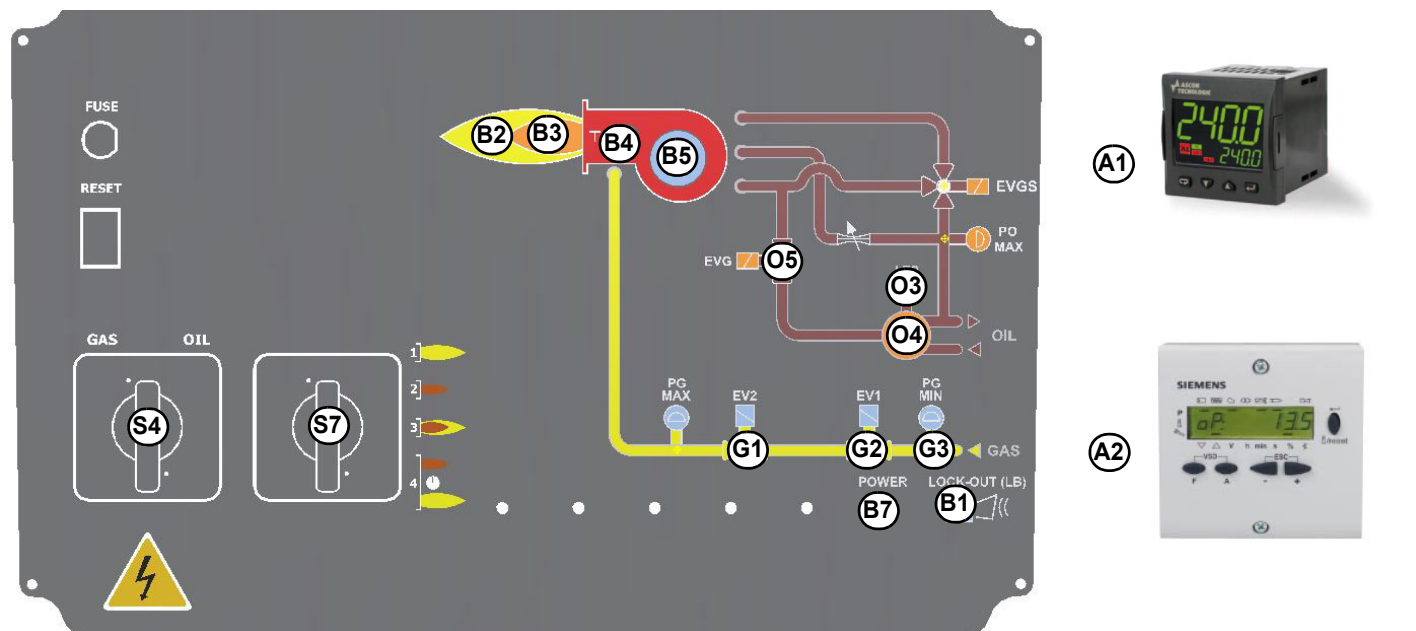
Рис. 8: передняя панель электрощита горелки
