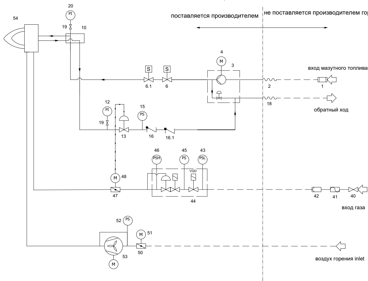
Fig. 1 - 3I2MG78 - Гидравлическая схема
