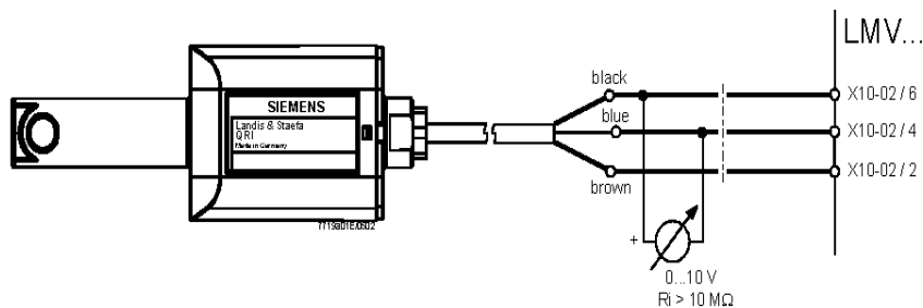
Рис. 9 - Детектирование с фотозлементом QRI..
