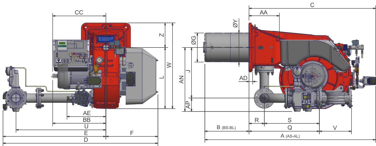
Flangia bruciatore
