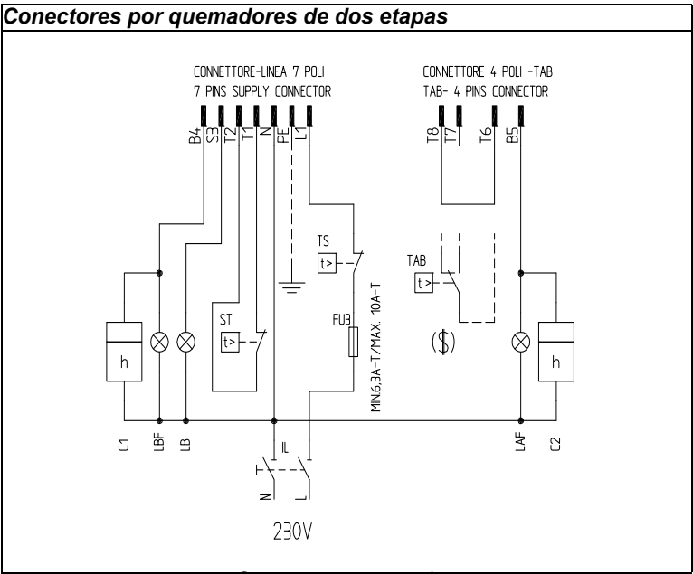
Conectores 7 y 4 polos
