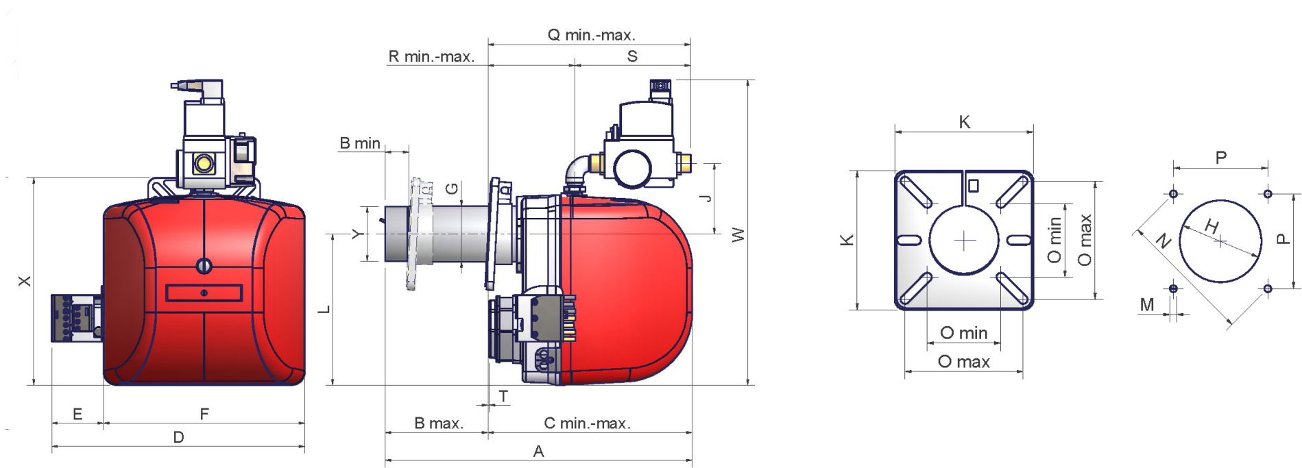
Brida quemador y plantilla de perforación de la placa de la caldera.
