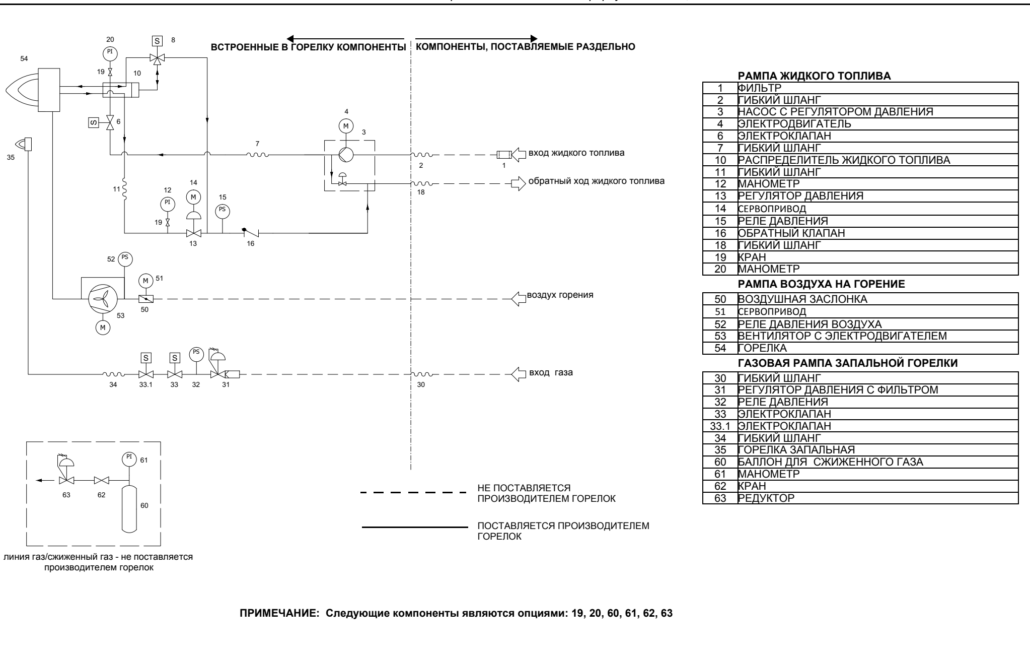
Рис. 5 - 3I2G-28 – Гидравлическая схема для форсунки типа G, KV
