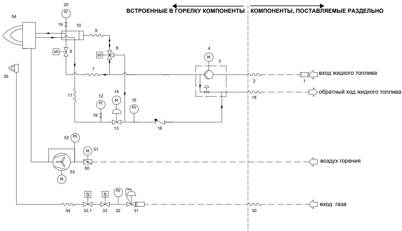
Рис. 4 - 3I2G-27 v0 – Гидравлическая схема для форсунки типа М3
