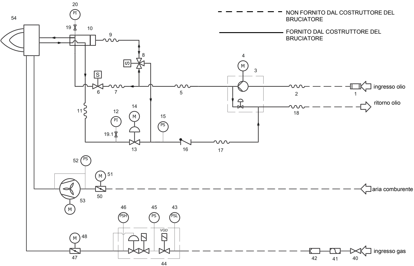
Fig. 2 - 3I2MG-23 v0 Schema idraulico
