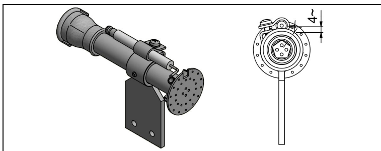
Рис. 16 Регулировка положения Электродов - Часть диффузора с запальной горелкой (Р) и запальным электродом (Е).
